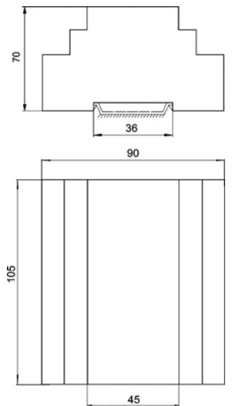
Рис. 1 Габаритные и установочные размеры БУАВР
